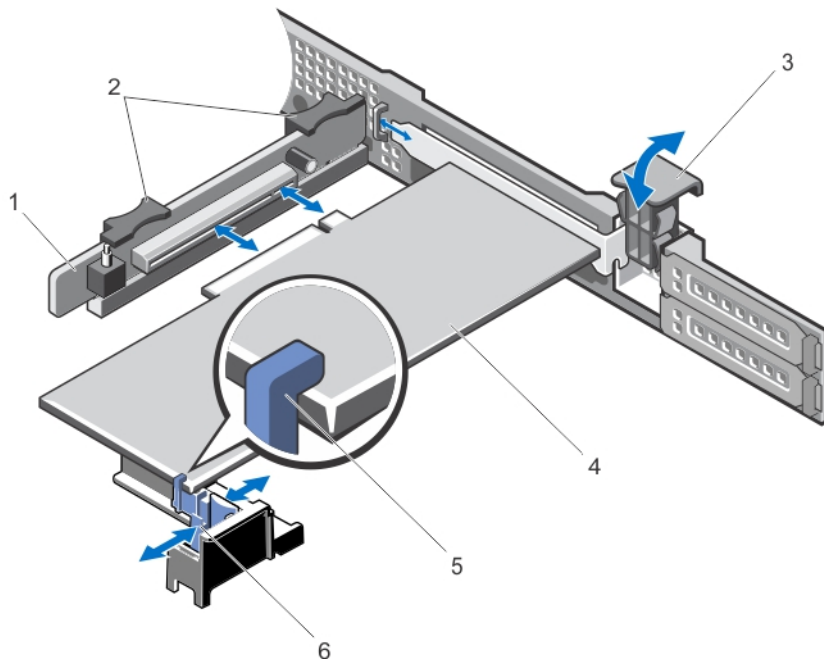
그림 21. 라이저 2에서의 확장 카드 분리 및 설치
