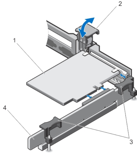
그림 20. 라이저 1에서의 확장 카드 분리 및 설치
