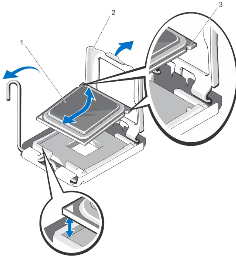
그림 29. 프로세서 분리 및 설치
