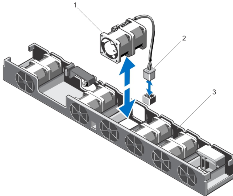
그림 18. 냉각 팬 분리 및 설치
