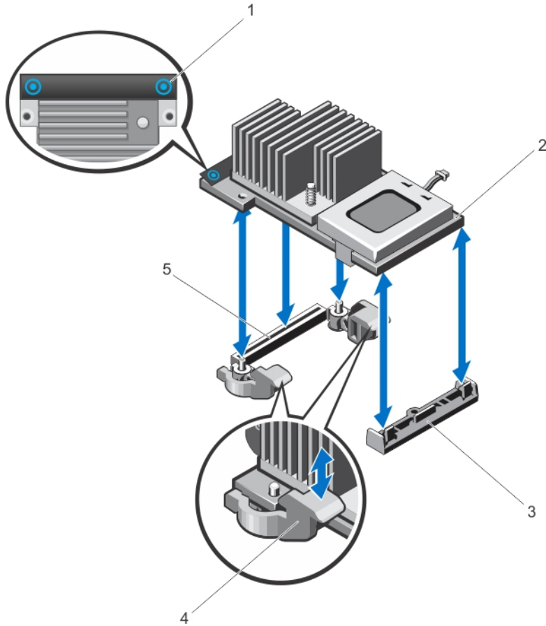
그림 27. 내장형 저장소 컨트롤러 카드 분리 및 설치
