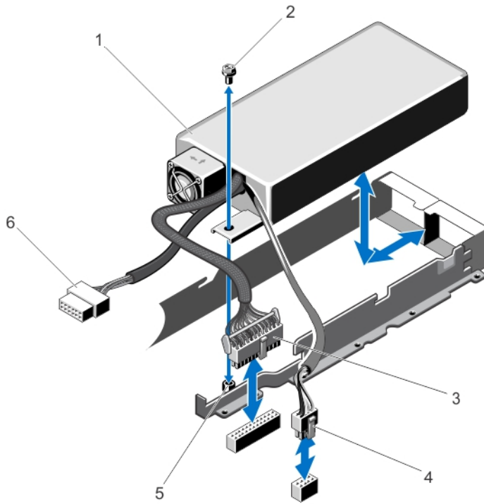
그림 31. 비중복 전원 공급 장치 분리 및 설치
