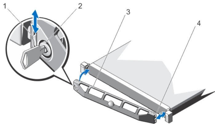
그림 8. 전면 베젤 설치 및 분리
