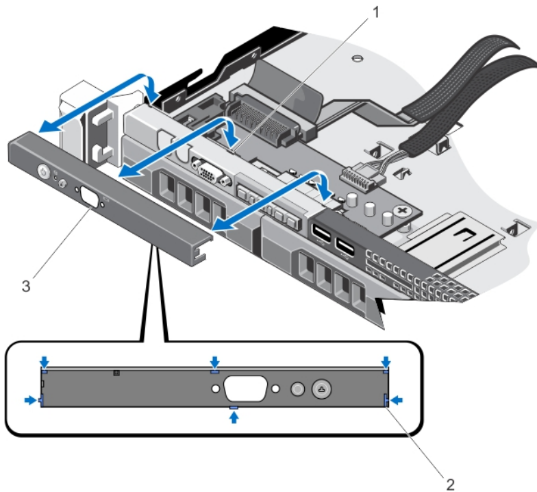
그림 38. 제어판 분리 및 설치
