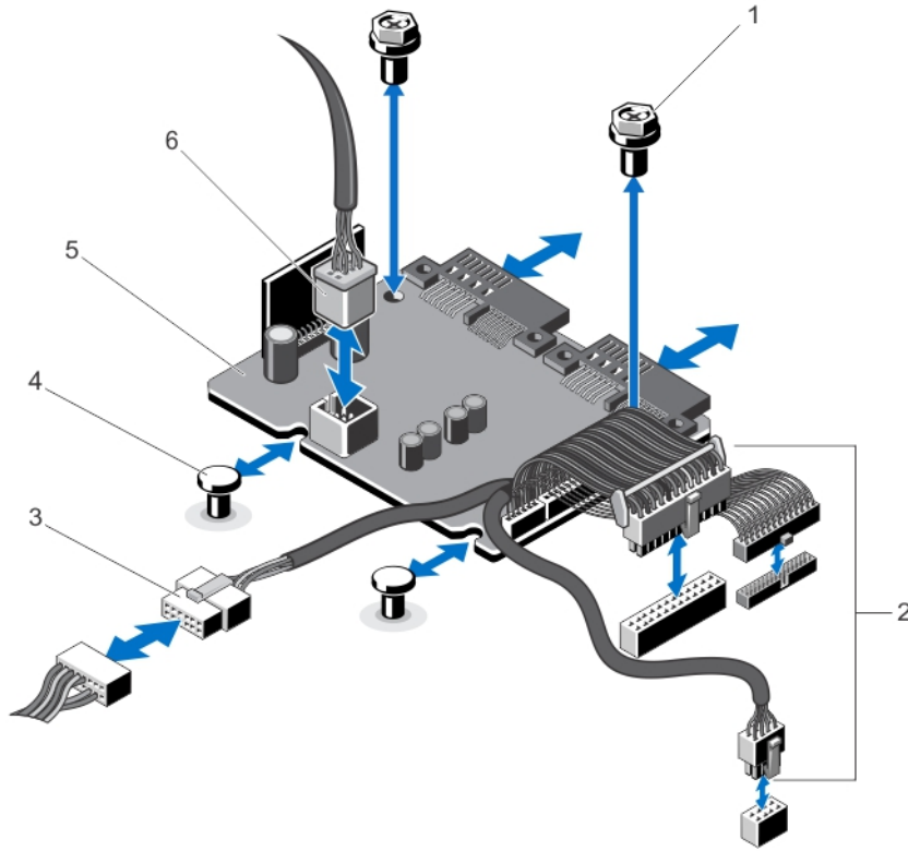
그림 41. 배전 보드 분리 및 설치
