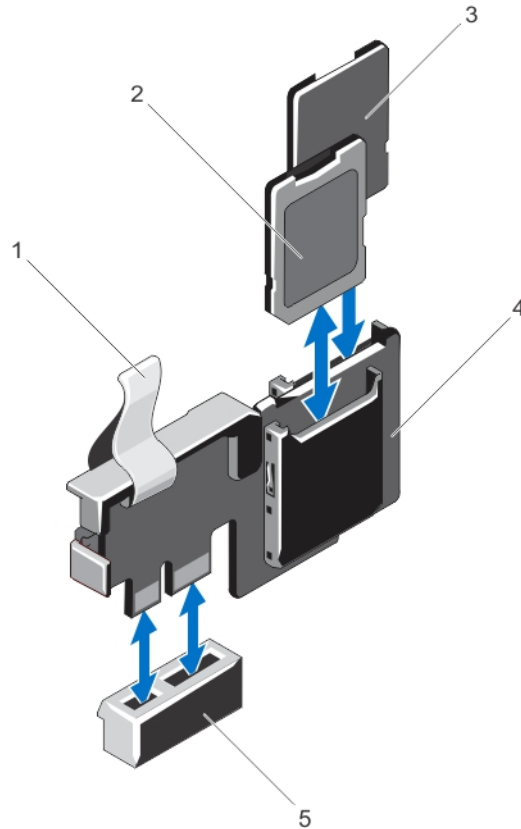
그림 26. 내부 이중 SD 모듈 분리 및 설치
