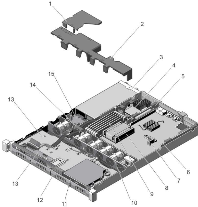
그림 10. 시스템 내부—중복 전원 공급 장치 포함
