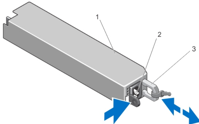
그림 30. 중복 전원 공급 장치 분리 및 설치
