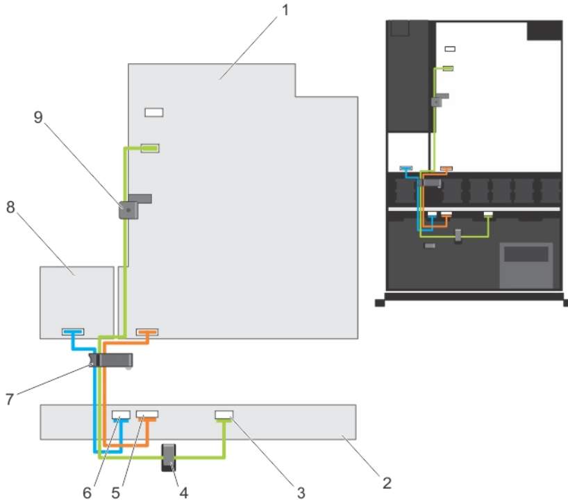
그림 37. 케이블 연결 다이어그램—4 개 하드 드라이브 후면판
