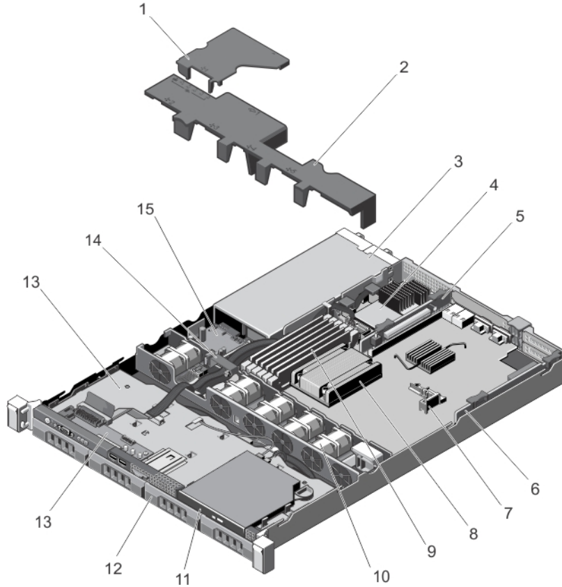
그림 11. 시스템 내부—비중복 전원 공급 장치 포함
