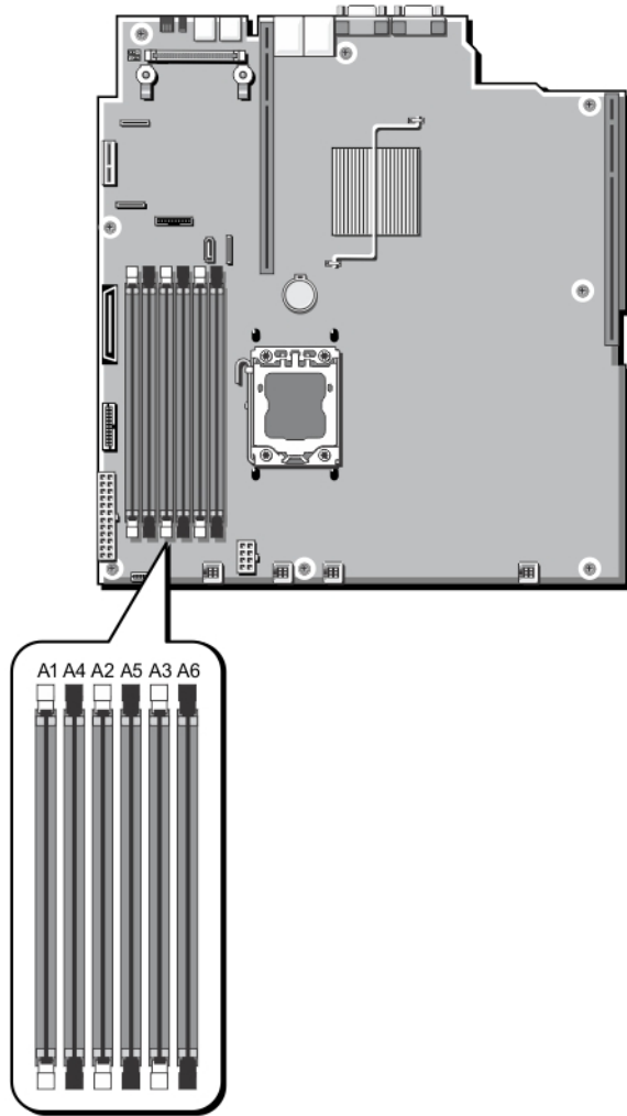
그림 13. 메모리 소켓 위치
