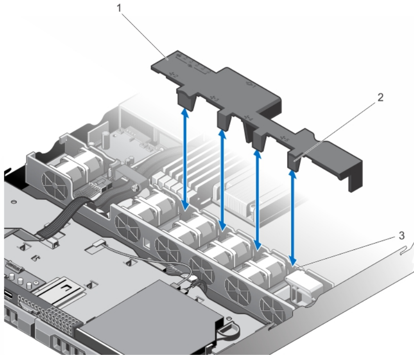
그림 12. 냉각 덮개 분리 및 설치
