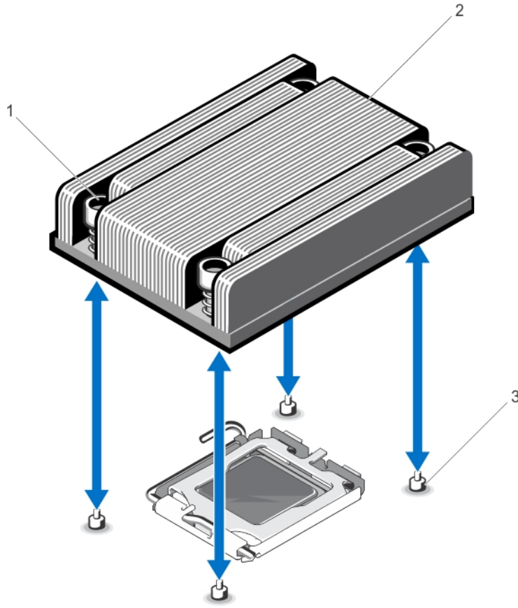
그림 28. 프로세서 방열판 분리 및 설치
