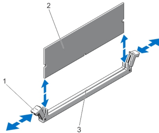
그림 14. 메모리 모듈 분리 및 설치
