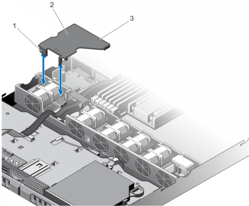
그림 40. PDB 덮개 분리 및 설치
