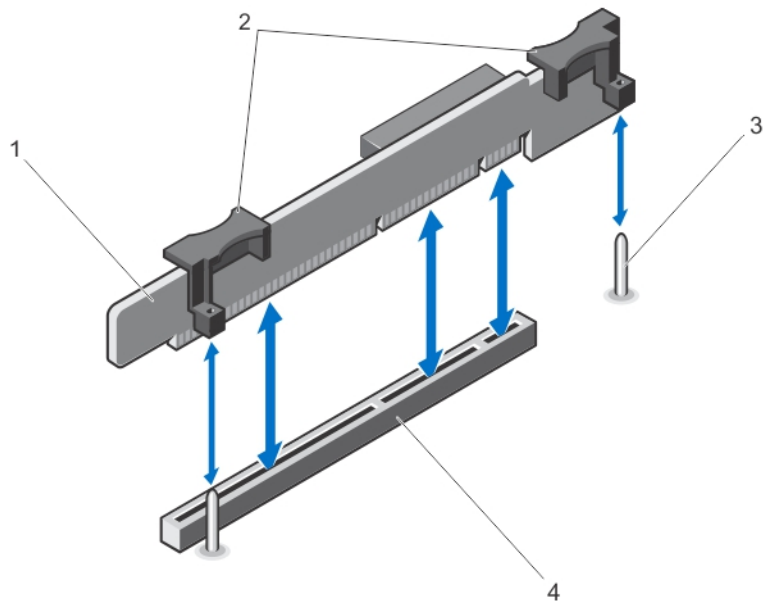
그림 22. 확장 카드 라이저 1 분리 및 설치
