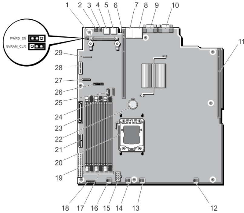
그림 43. 시스템 보드 점퍼 및 커넥터
