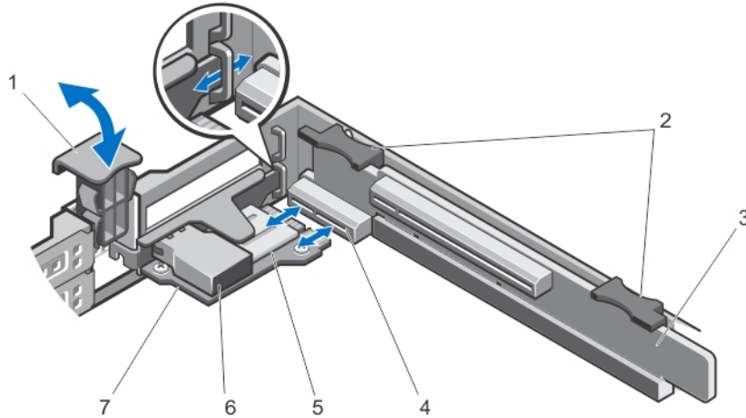
그림 24. iDRAC Ports 카드 분리 및 설치
