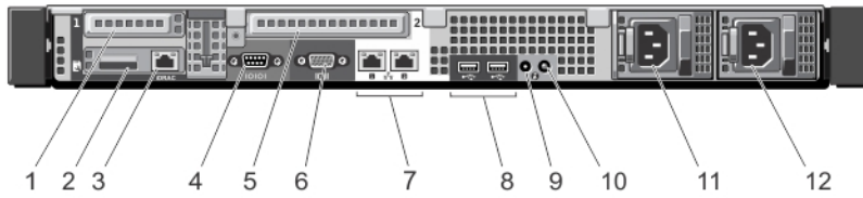
그림 4. 후면 패널 구조 및 표시등 —(중복 전원 공급 장치 포함)
