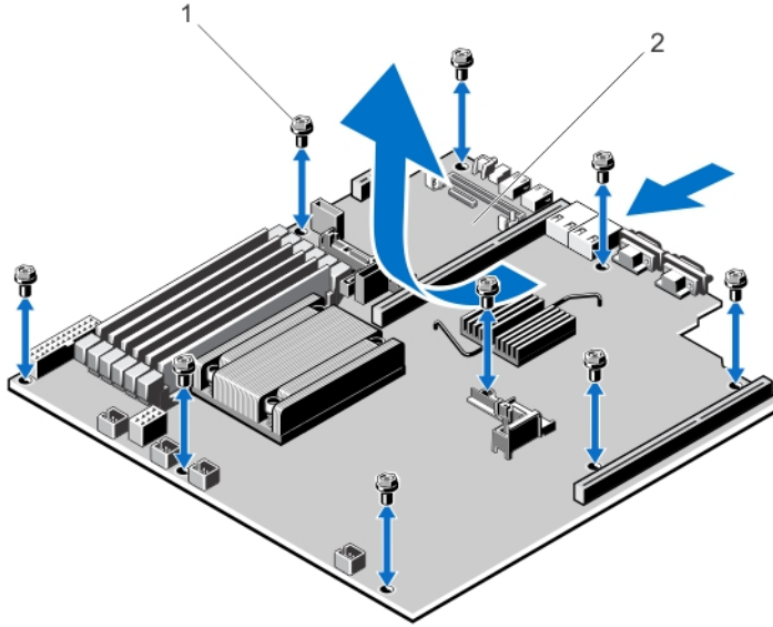
그림 42. 시스템 보드 분리 및 설치
