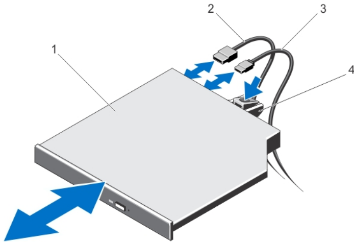
그림 17. 광학 드라이브 분리 및 설치(핫 스왑 가능한 하드 드라이브 시스템)
