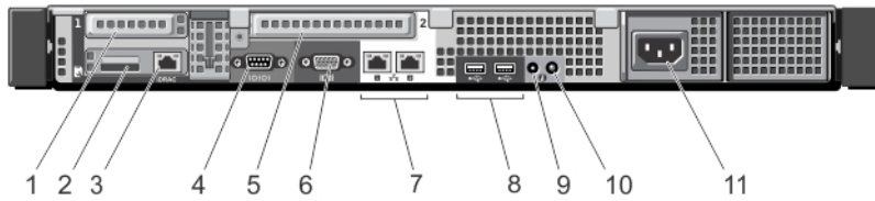
그림 5. 후면 패널 구조 및 표시등 —(비중복 전원 공급 장치 포함)
