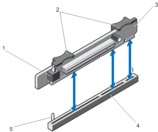
그림 23. 확장 카드 라이저 2 분리 및 설치
